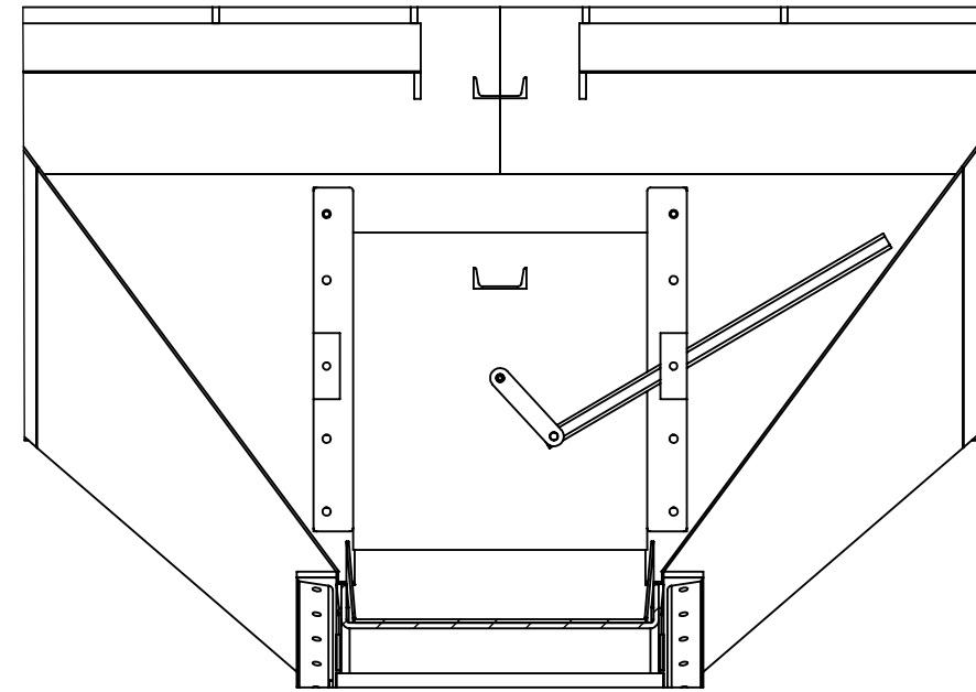
SECTION A-A ADJ. DOOR ASSEMBLY SCALE 1 : 16
